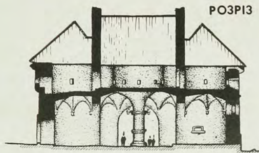
РОЗРІЗ
